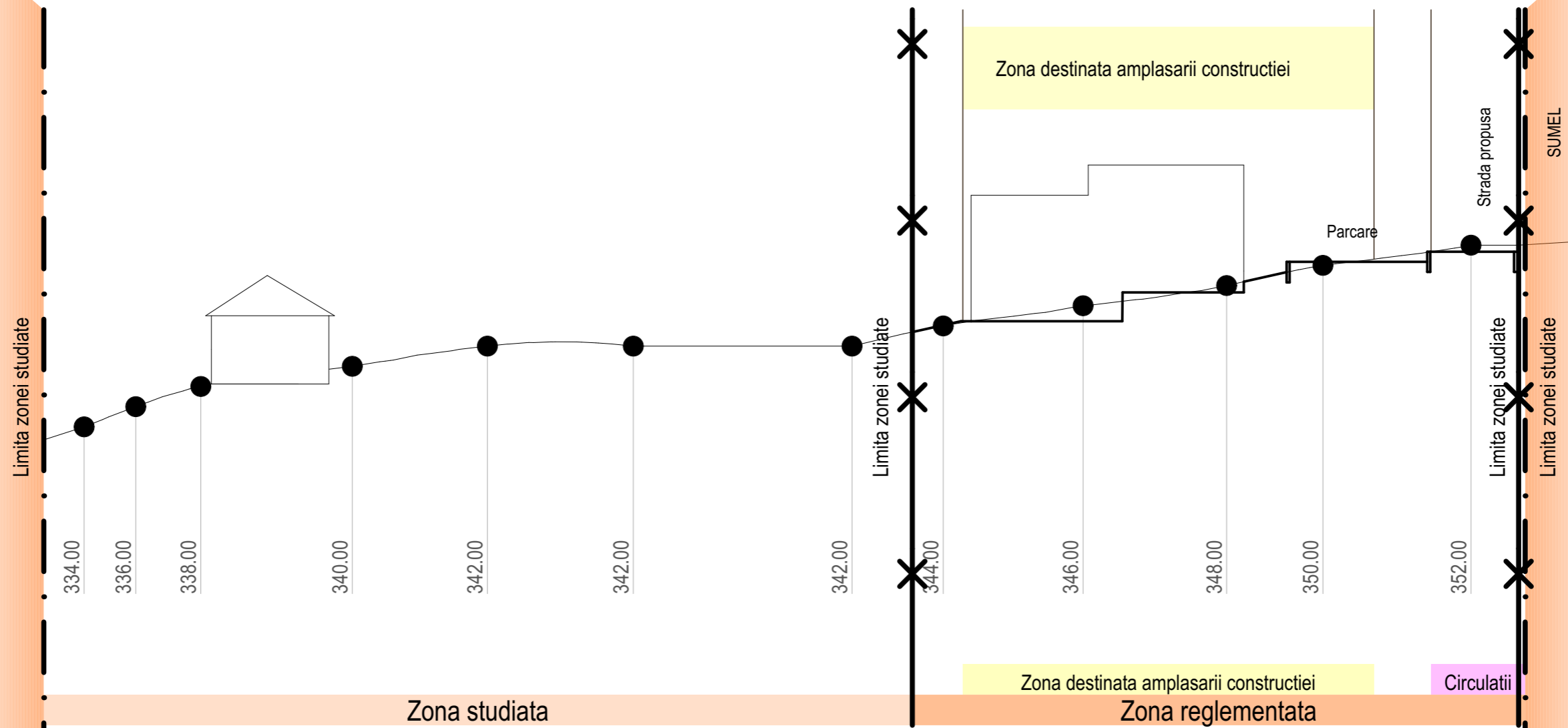
Profil strada Scara 1:200
